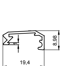
5036 0,108 Kg/m
