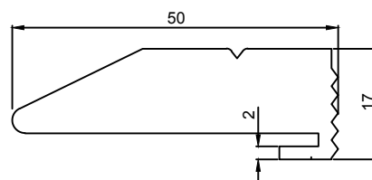
5049 1.525 Kg/m
