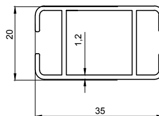
5041 0,405 Kg/m
