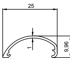
5015 0,103 Kg/m
