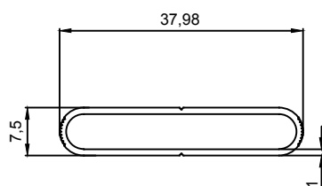
5048 0,216 Kg/m
