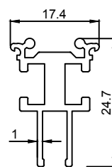
5002 0.330 Kg/m
