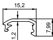
5017 0,084 Kg/m
