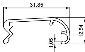
5012 0.208 Kg/m
