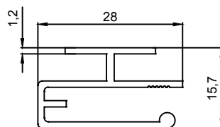
5027 0,300 Kg/m
