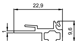
5000 0.148 Kg/m
