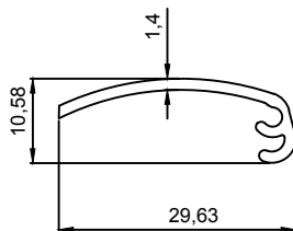
5024 0,154 Kg/m
