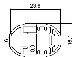
5025 0.245 Kg/m
