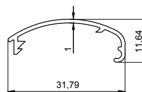
5038 0,138 Kg/m
