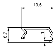
5016 0,089 Kg/m
