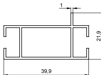
5051 0,354 Kg/m
