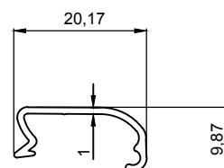
5031 0,102 Kg/m
