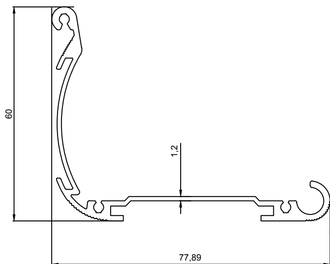
5045 0,778 Kg/m
