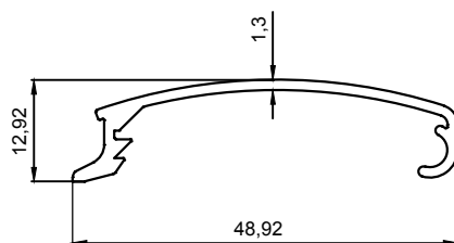
5037 0,275 Kg/m
