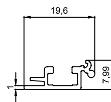
5005 0,119 Kg/m
