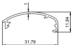
5032 0,138 Kg/m
