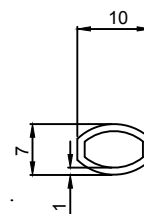
5028 0,068 Kg/m
