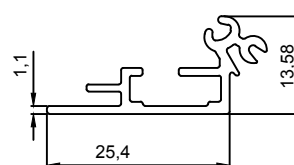
5008 0.222 Kg/m
